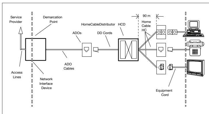
Das NK HomeNet im schematischen Überblick mit den darauf realisierbaren Diensten.
